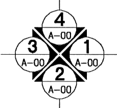
แปลนโครงหลังคา มาตราส่วน 1:125
